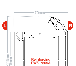
Transom Z EWS 7703
