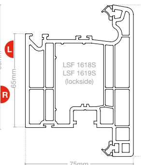
Door sash T LSF 1019
