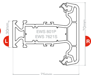
Transom T LSF 1002
