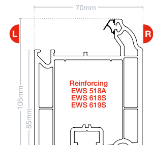
Door sash Z EWS 7718
