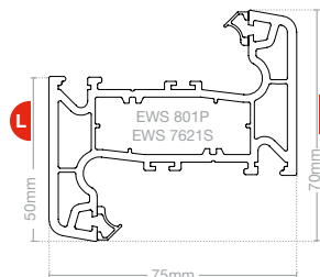
Transom Z LSF 1003
